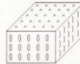
Struktura Smectická
