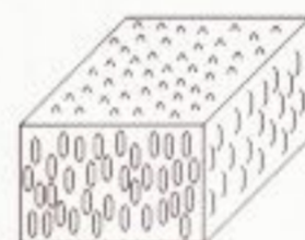
Struktura Nematická
